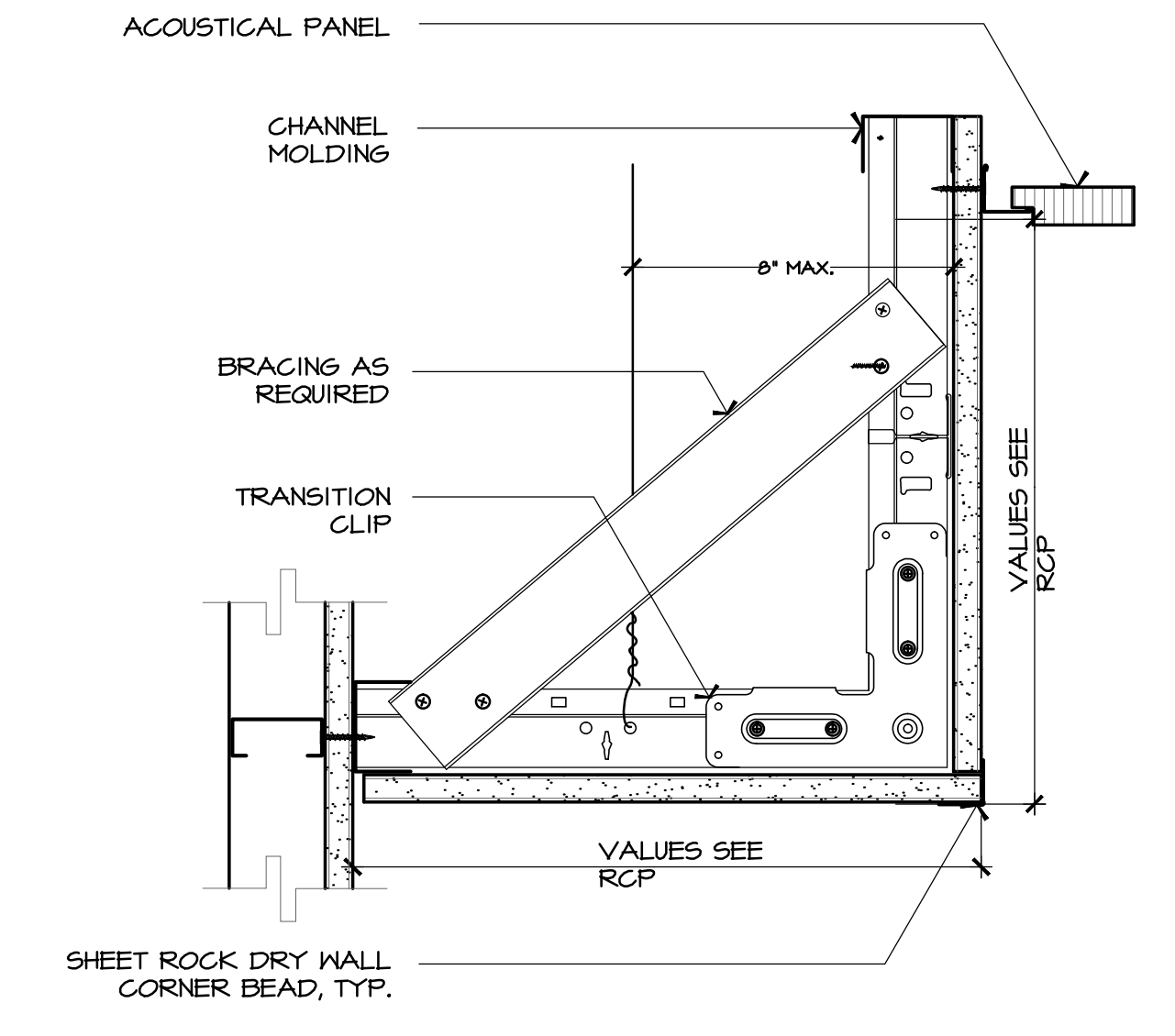
10 SOFFIT & ACOUSTICAL DET. CLG-SOFFIT AND ACOUSTICAL TRANSITION.DWG SCALE: N.T.S.
