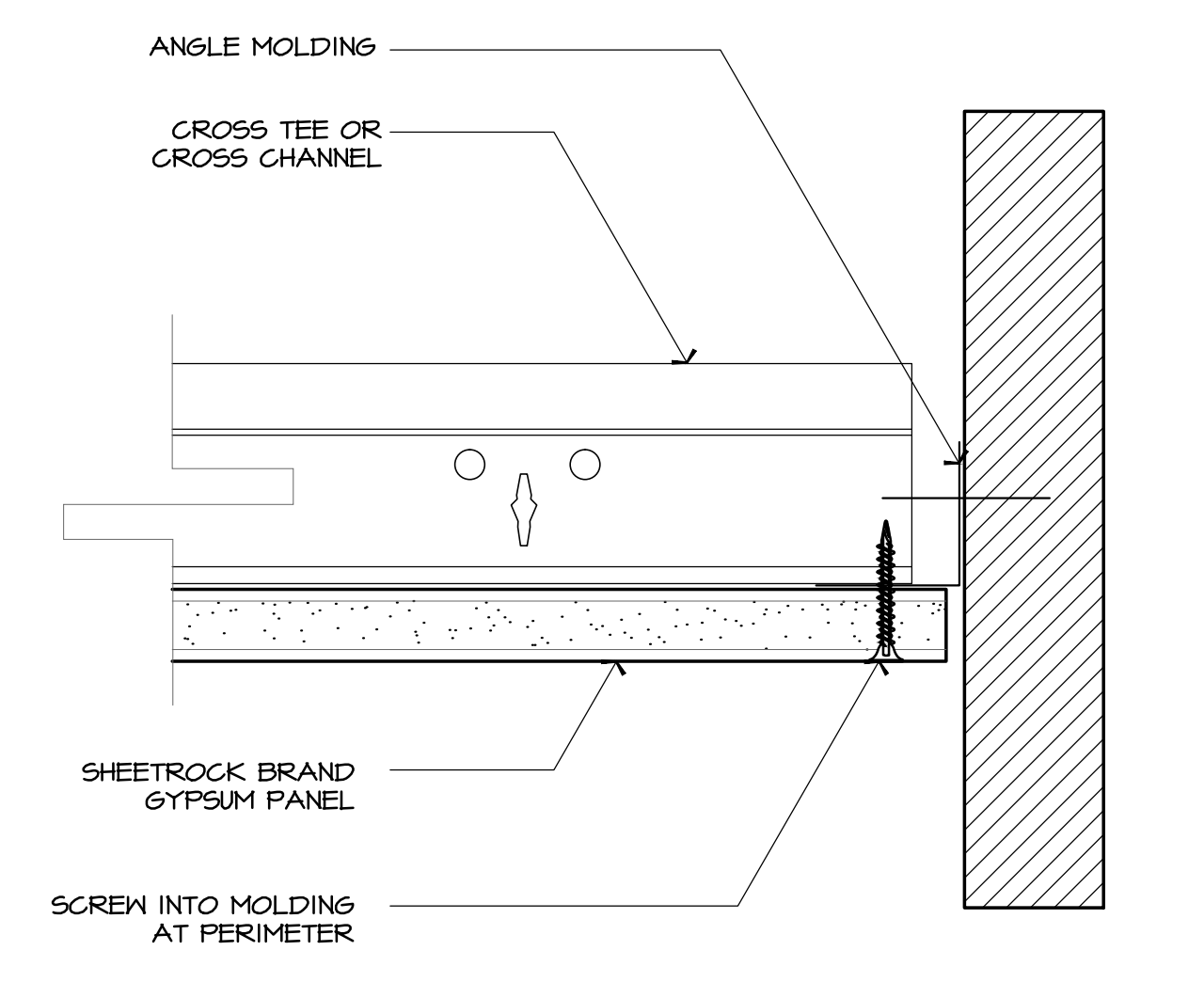
8 ANGLE MOLDING DETAIL CLG-ANGLE MOLDING.DWG SCALE: N.T.S.
