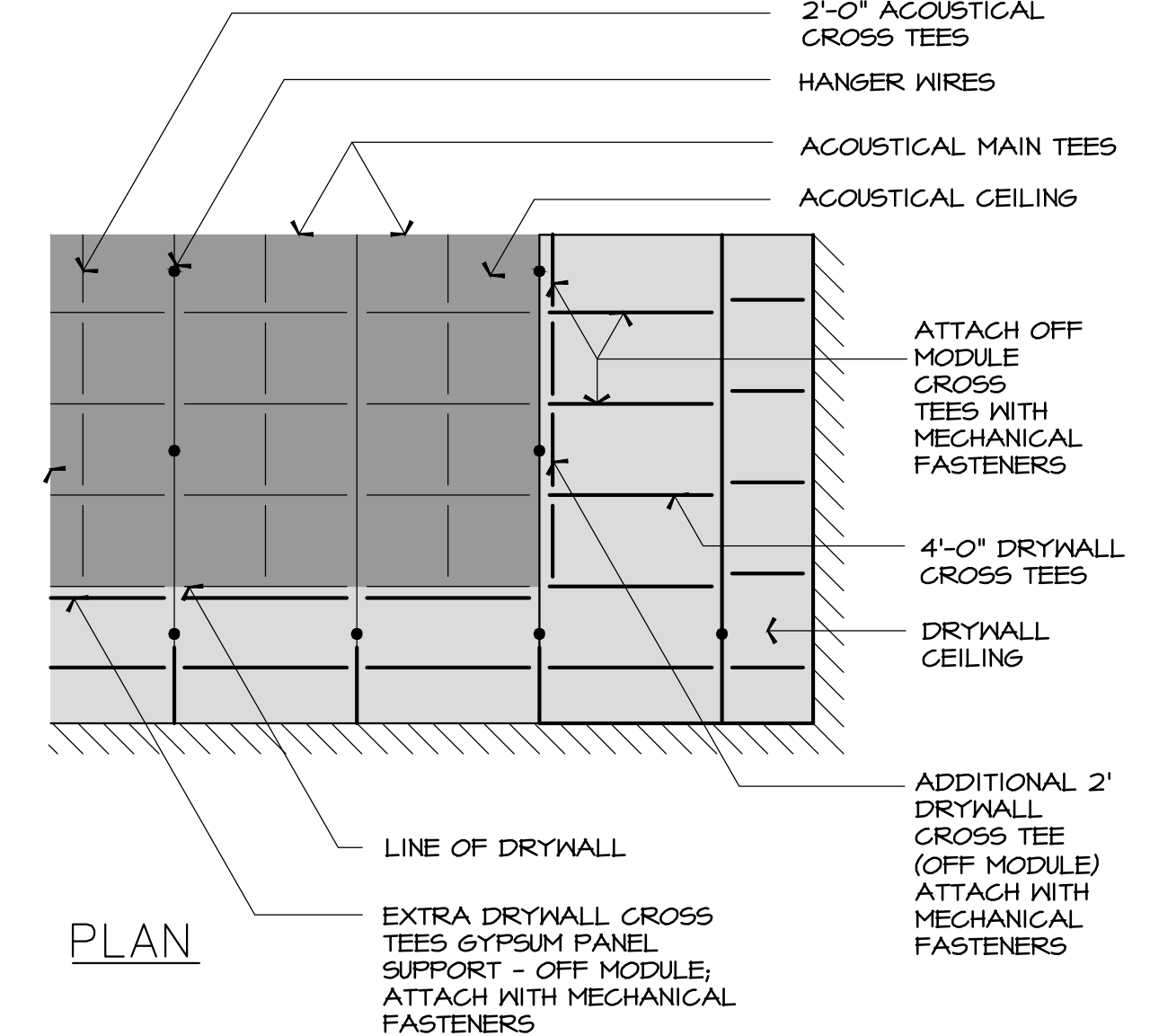
7 DRYWALL-ACOUSTICAL TRANS. CLG-PLAN VIEW.DWG SCALE: N.T.S.
