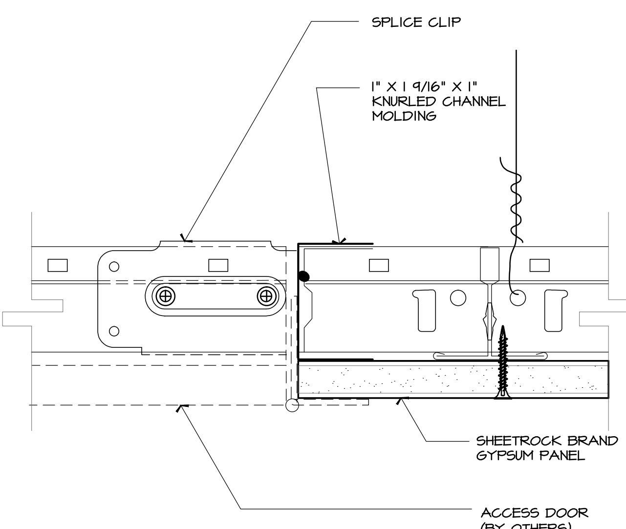
5 ACCESS DOOR DETAIL CLG-ACCESS DOOR.DWG SCALE: N.T.S.
