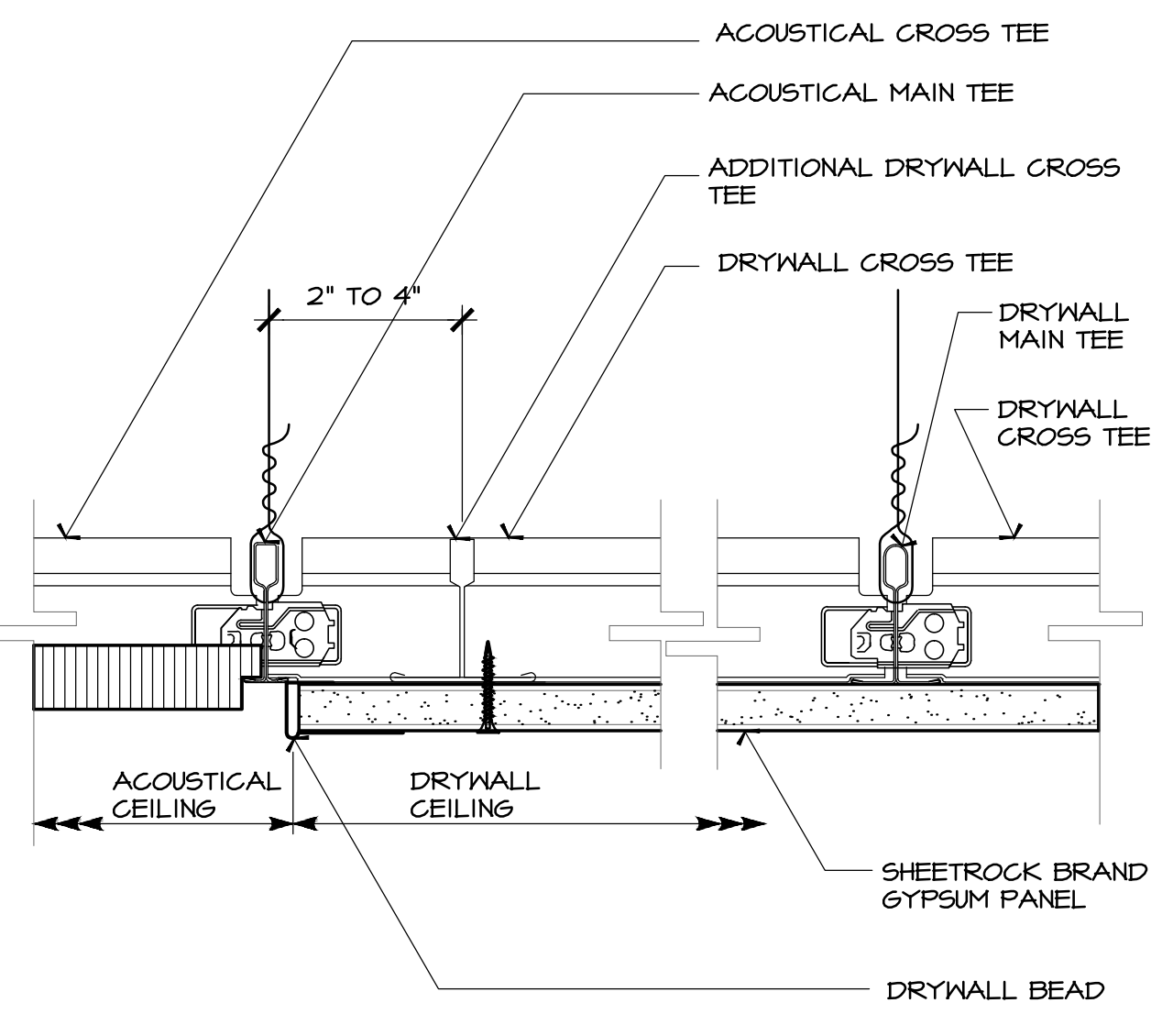
9 DRYWALL - ACOUSTICAL DET. CLG-DRYWALL-ACOUSTICAL TRANSITION.DWG SCALE: N.T.S.
